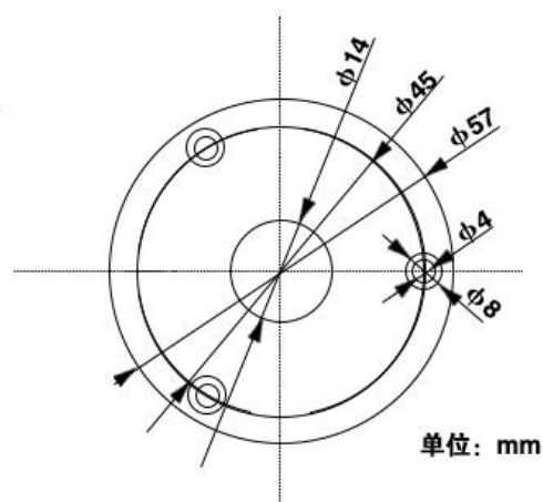
用螺丝将法兰盘固定在排风管上
