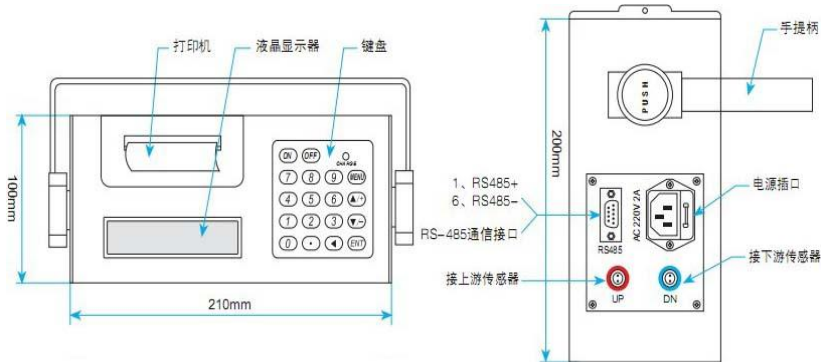
外形尺寸及接线图
