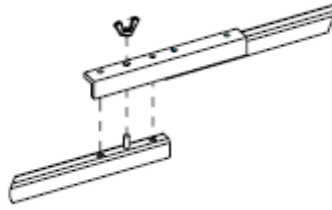
图 20 框架边缘连接装配结构
