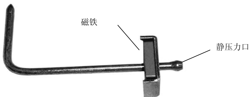
图 9： 静压探针
