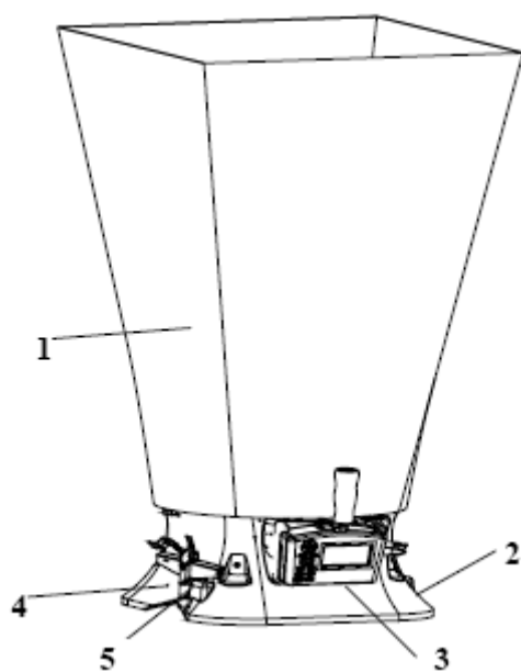
图 13 风罩的组成
