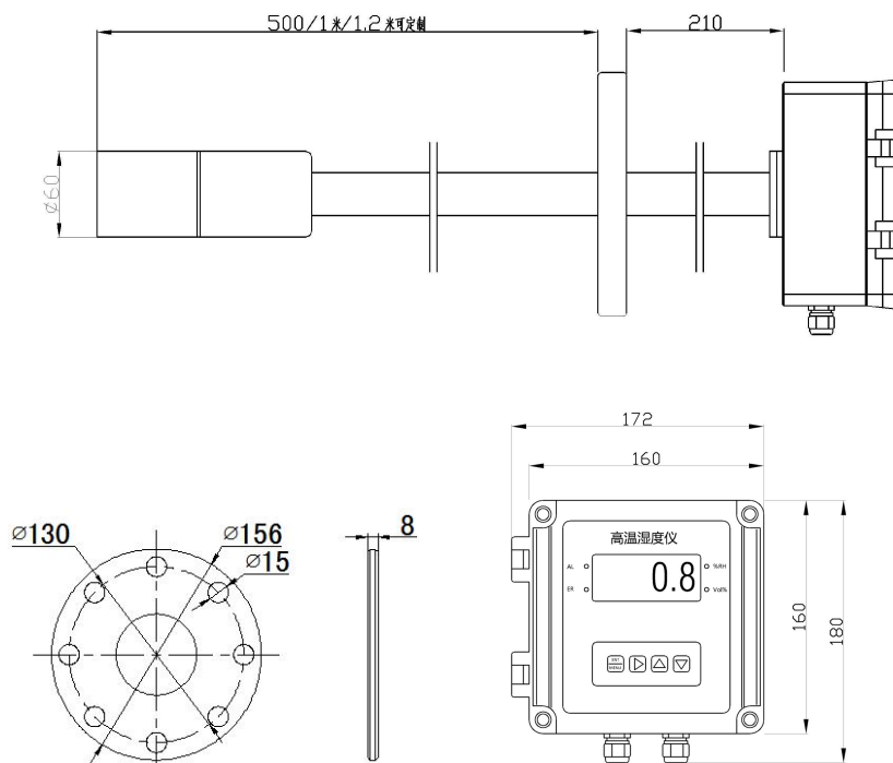
安装法兰尺寸图
