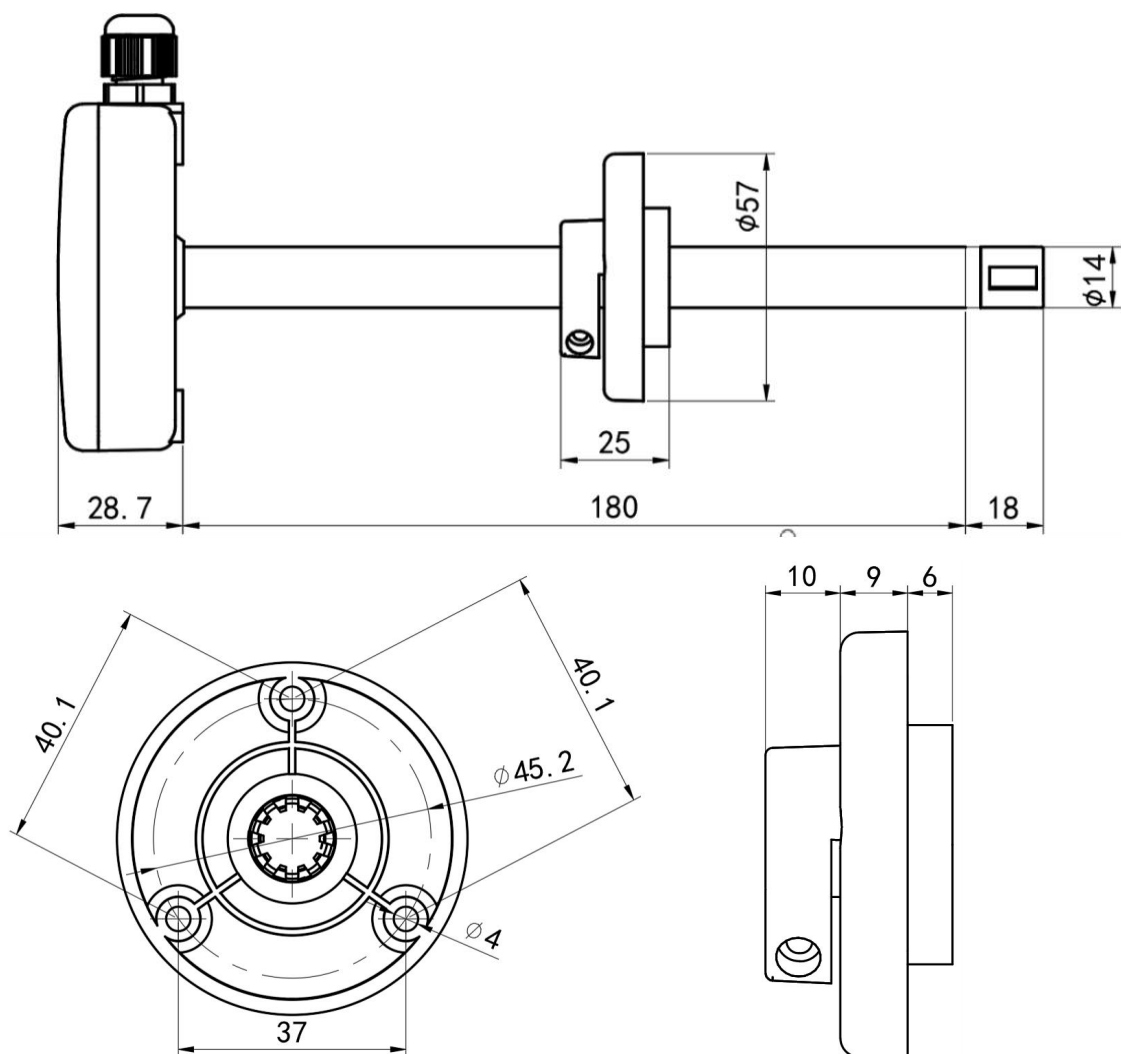
壳体尺寸
