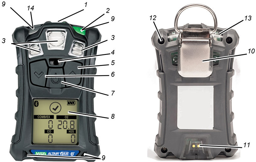
图 1 产品概述
